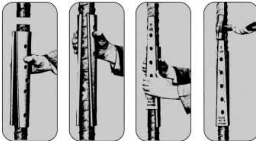
G-Loc®-Klemmen für Betonstahl nach DIN 488
